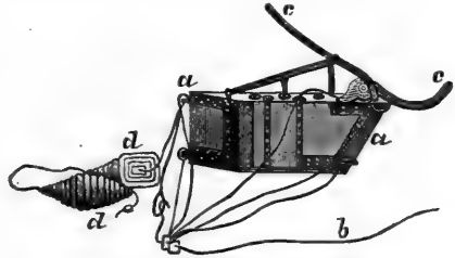
FIG. 2.—HARVEY TORPEDO.
